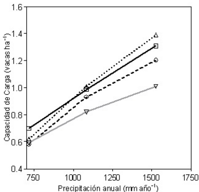
Figura 3: Respuesta en la capacidad de carga ante años contrastantes de precipitación anual, en cada una de las cuatro unidades funcionales descriptas. Para el cálculo de la capacidad de carga se utilizó la ecuación genérica: Capacidad de Carga = (PPNA x IC) / CI. El Consumo Individual, CI, se estimó como el 3% del peso vivo, en un animal de 400 kg de peso vivo, esto representa 12 kg MS.día -1 . El índice de cosecha, IC, se calculó a partir de la ecuación propuesta por Golluscio et al (1998): IC = -5.51 + 0.7154 \times (PPNA)^{0.5} .
